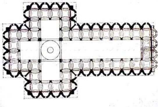
Ilustración 22. Planta original.
