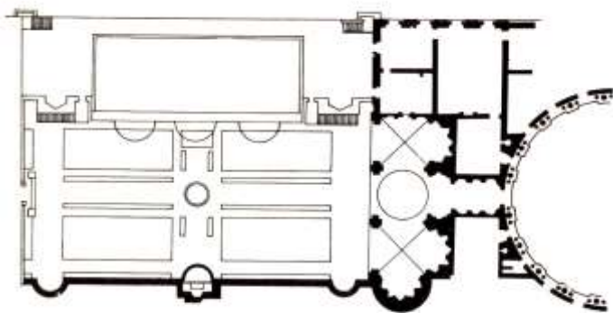
Planta de la Villa Madama, en Roma, construida por Rafael hacia 1516
