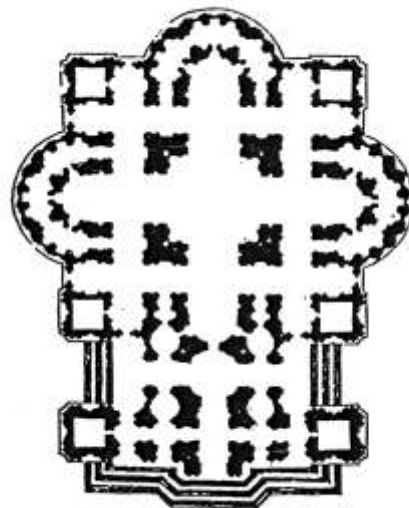
Ilustración 141. Proyecto de San Pedro de Sangallo.
