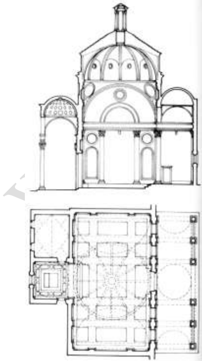
Ilustración 30. Alzado y planta.
