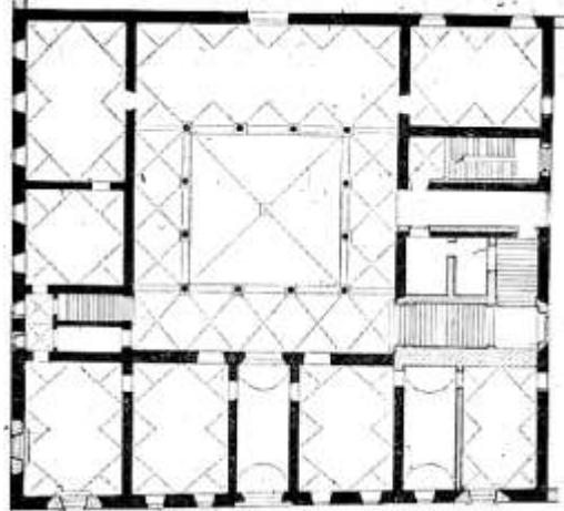
Ilustración 39. Planta Palacio Medici-Riccardi.
